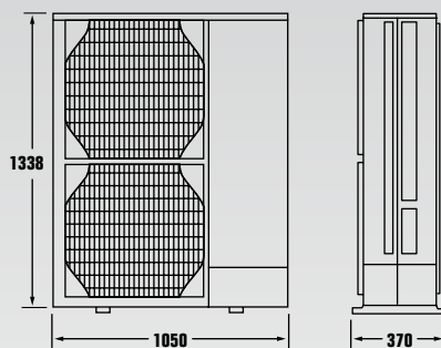
Buitenunit ODU 10/11/12
