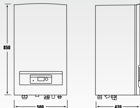
Binnenunit
