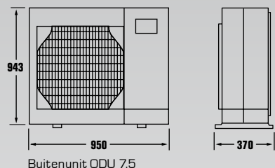
Buitenunit ODU 7,5
